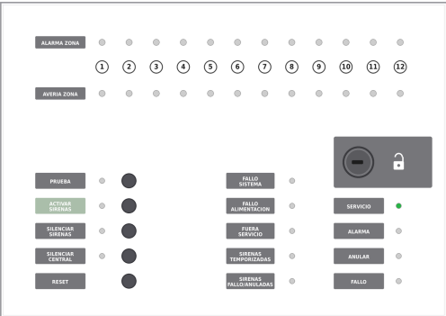
Frontal de la central (esquema A2J según el manual del fabricante)
